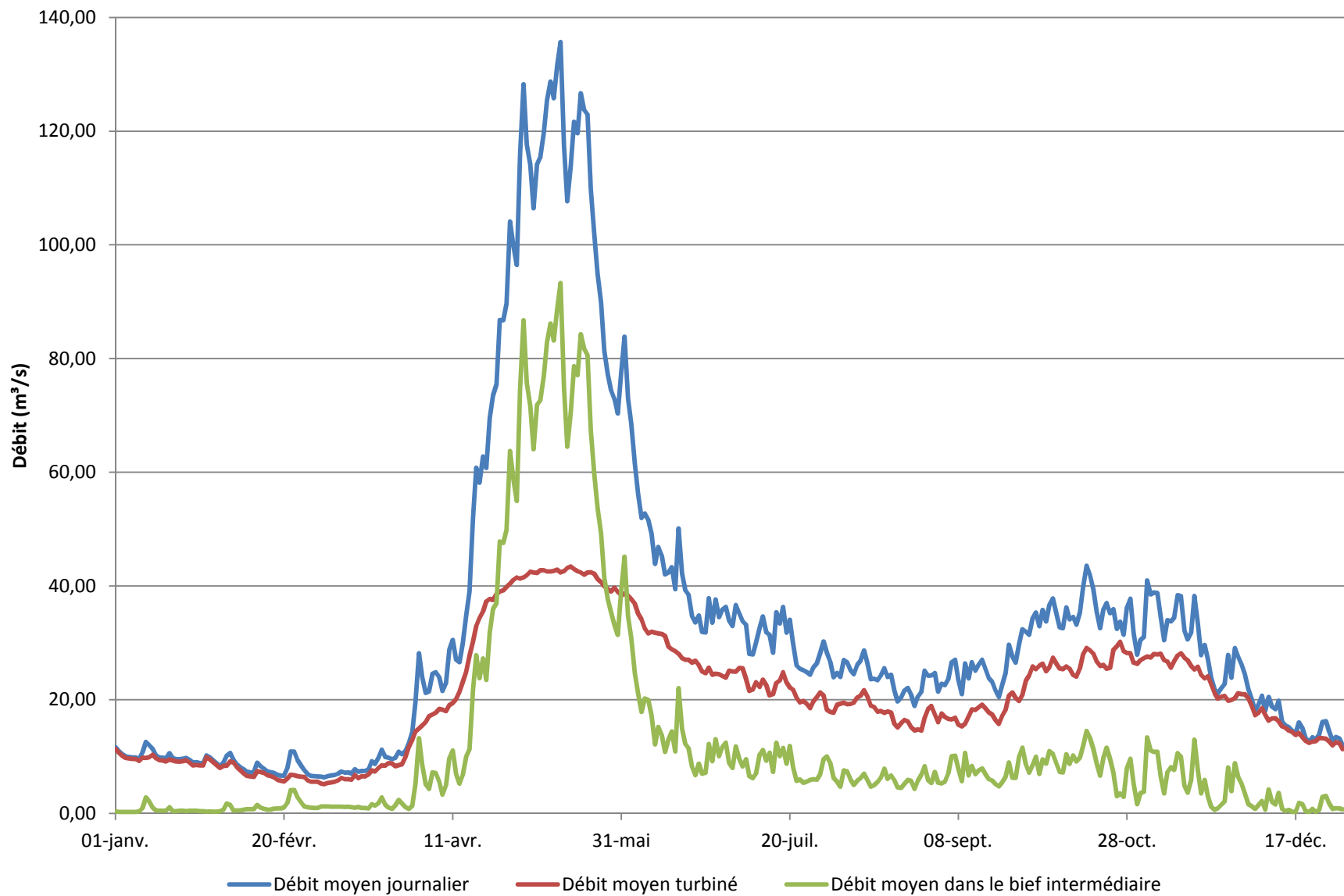
Figure A-5 : Distribution des débits moyens journaliers pour le bief intermédiaire du projet HCSJ
